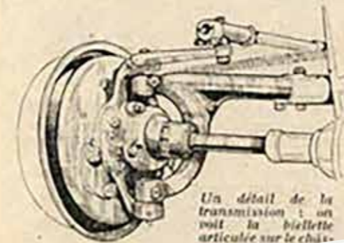
Un détail de la transmission : on voit la biellette articulée sur le châssis et le double débraillement de la roue. La voiture est bien dégagée grâce à la suspension spéciale qui est une adaptation aux roues avant motrices de l'ancien système Dailia, c'est-à-dire un cantilever longitudinal de chaque côté, avec, à chaque bout une biellette articulée supportant les roues.
